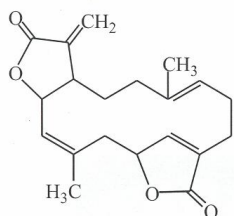
Ovatodiolide
