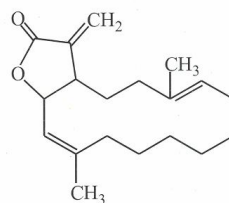
Anisomelolide
