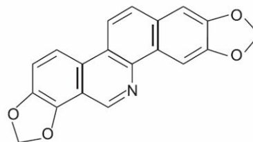
Norsanguinarine
