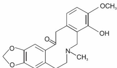
Hunnemanine
