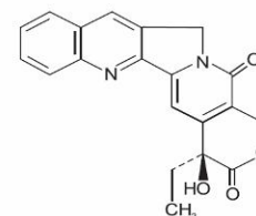
Camptothecin
